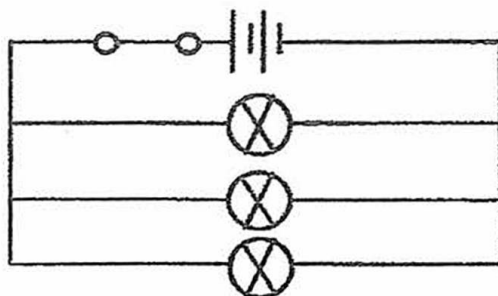
Circuit Y
